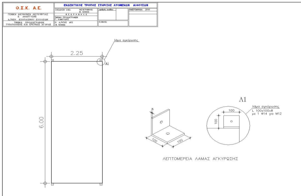
Σχέδιο ενδεικτικού τρόπου στήριξης λυόμενων αιθουσών
