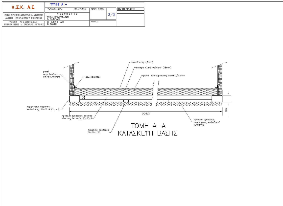
Συμπληρωματικά Σχέδια – Σχέδιο 2
