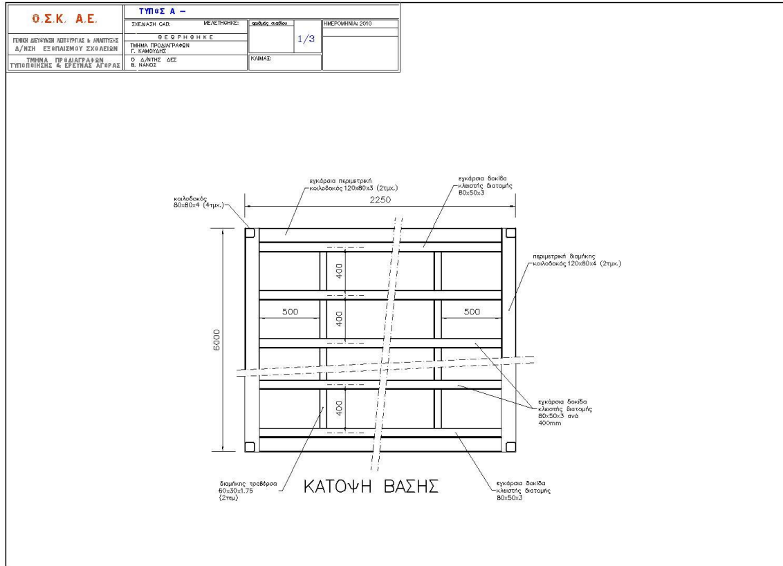
Συμπληρωματικά Σχέδια – Σχέδιο 1
